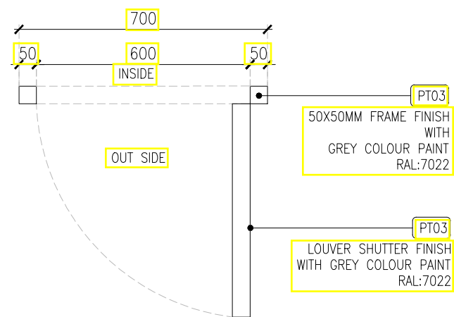
PLAN (LD)
