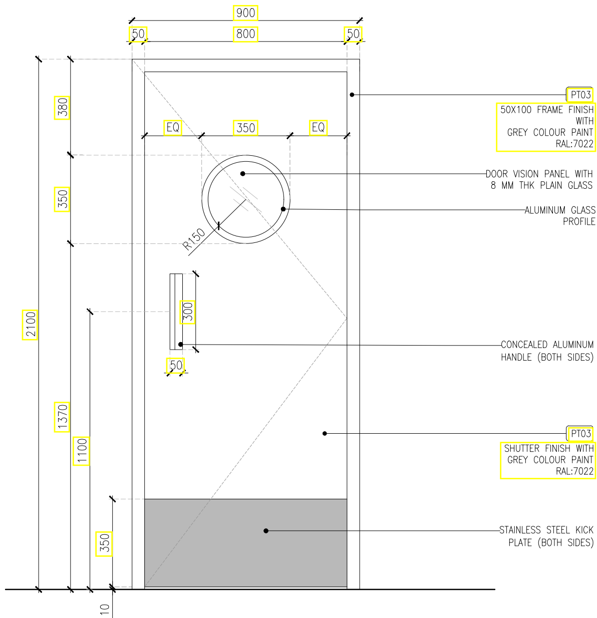
ELEVATION (D)
