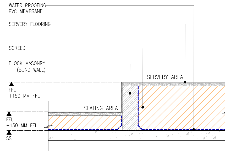
SECTION-A (SCALE 1:10)
