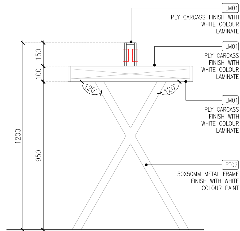
SECTION-A (SCALE-1:15)
