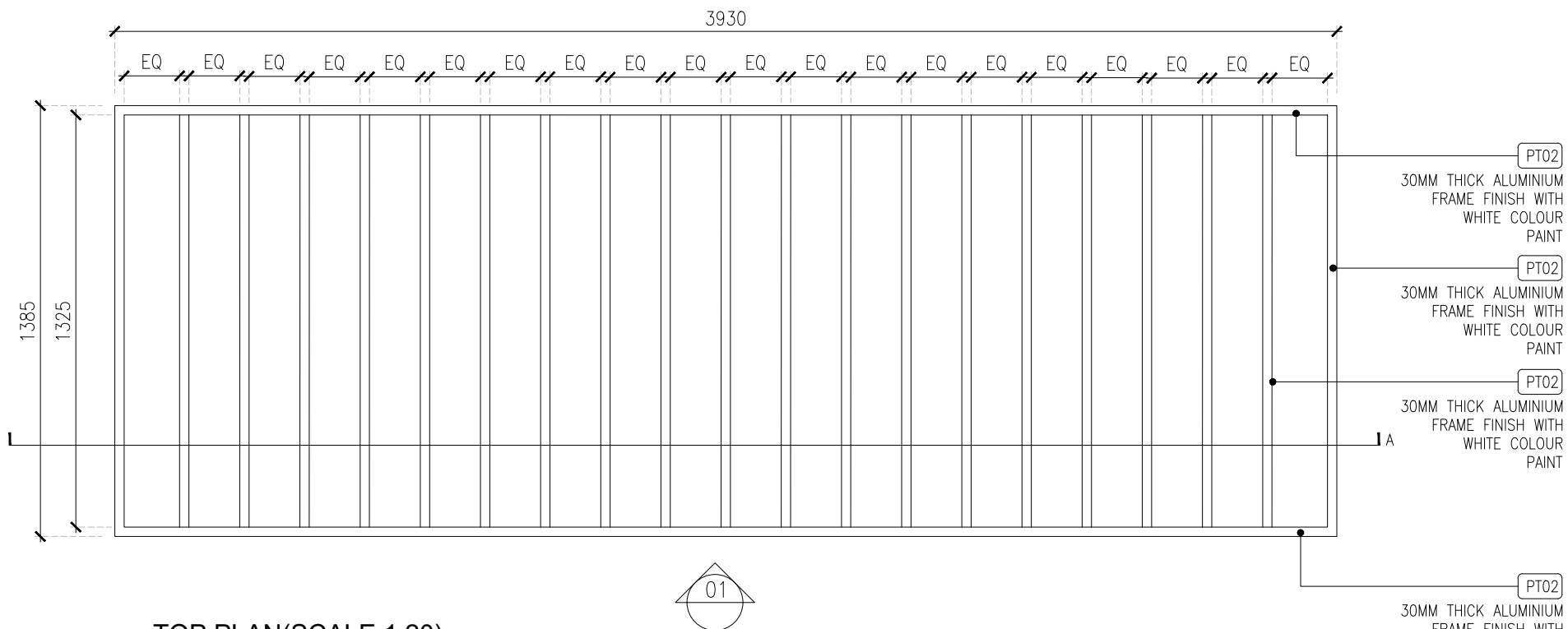
TOP PLAN(SCALE 1:20)
