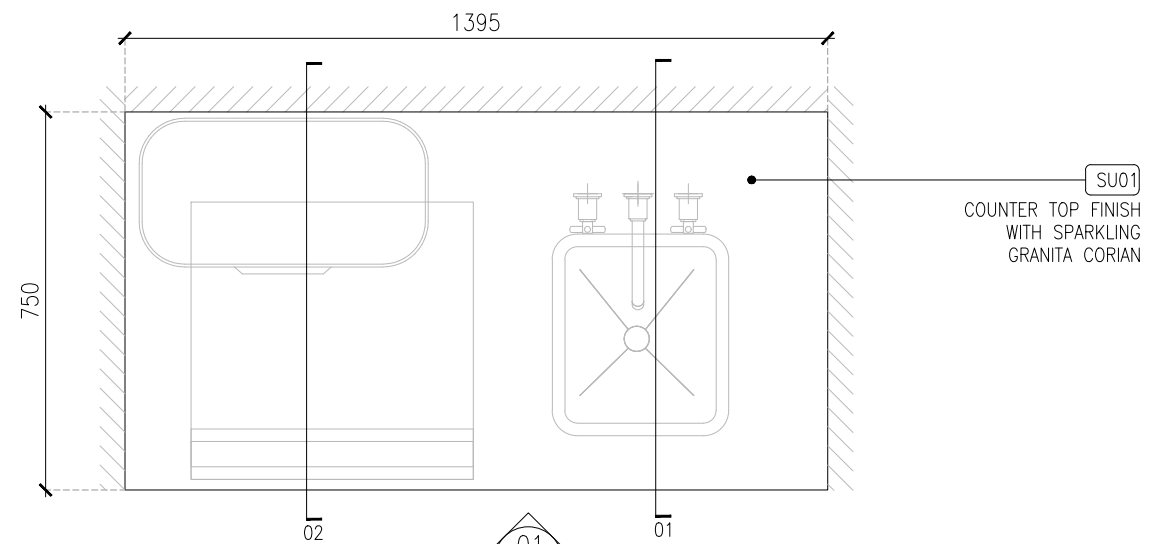
TOP PLAN (SCALE 1:15)
