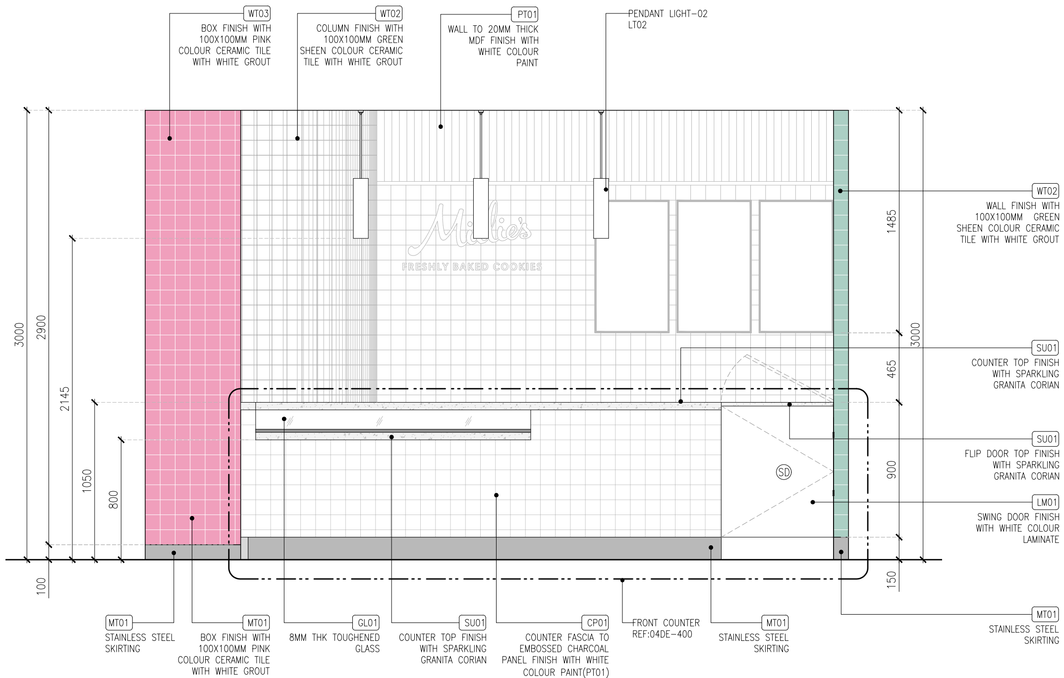
01 ELEVATION - 03 03IL-302 1:25
