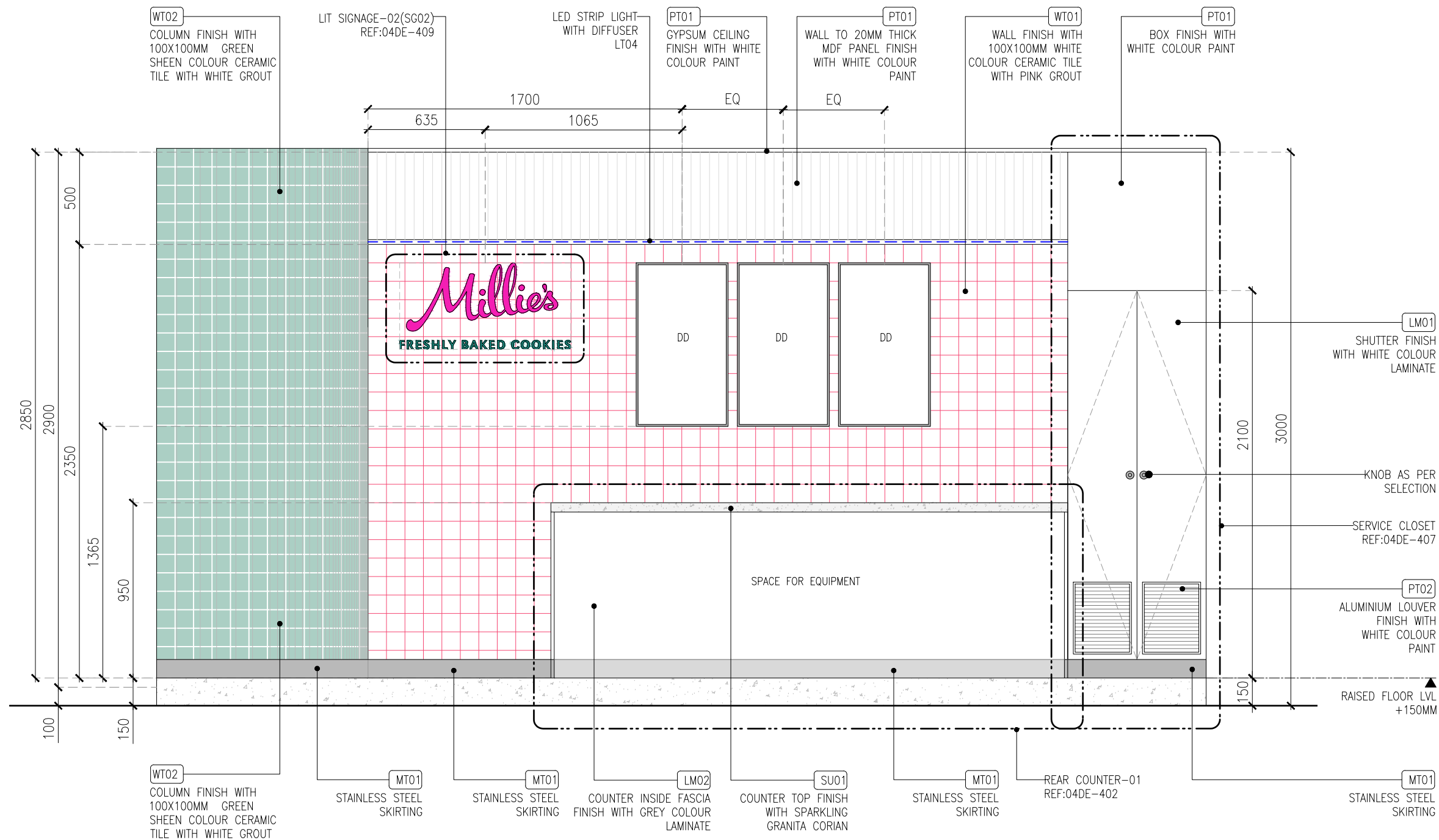
01 ELEVATION-04 03IL-303 1:25
