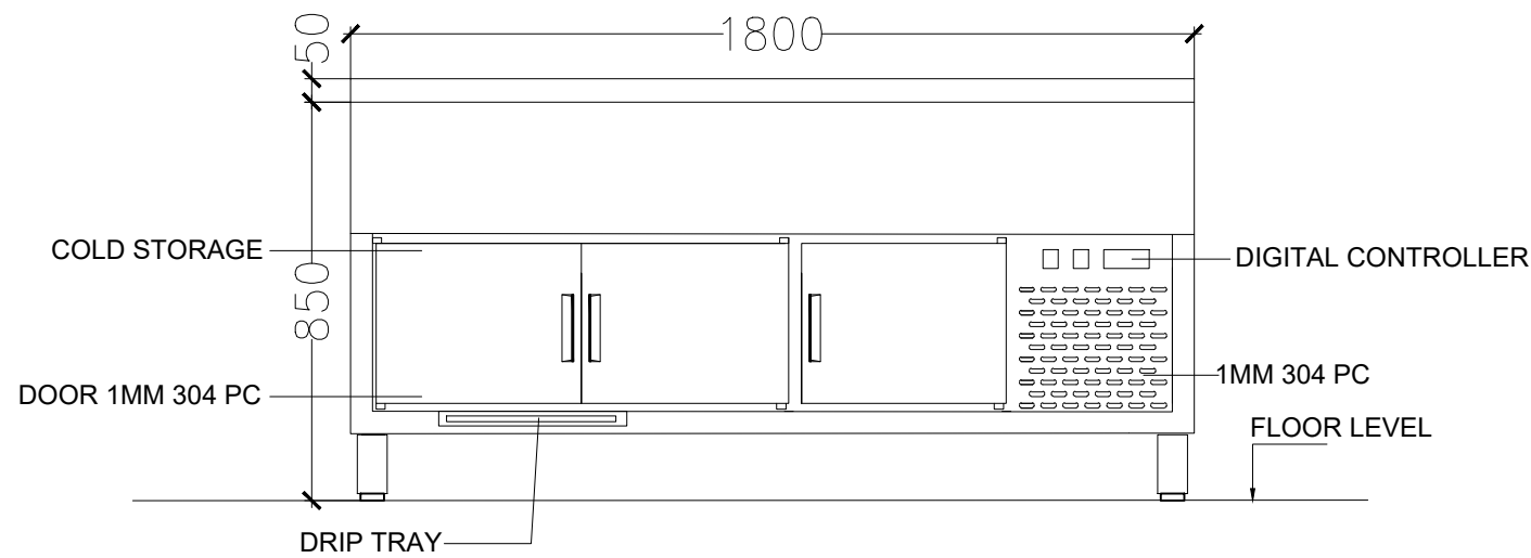
ELEVATION A-A
