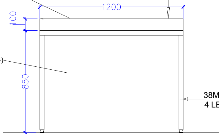
ELEVATION A
