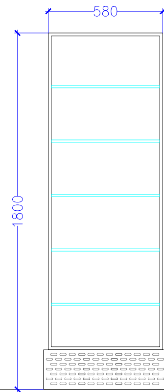
ELEVATION A
