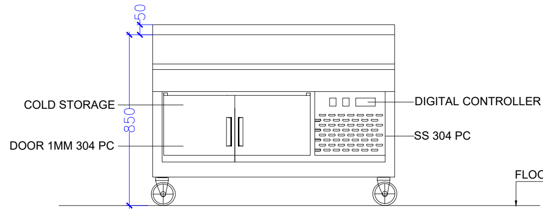
ELEVATION A-A
