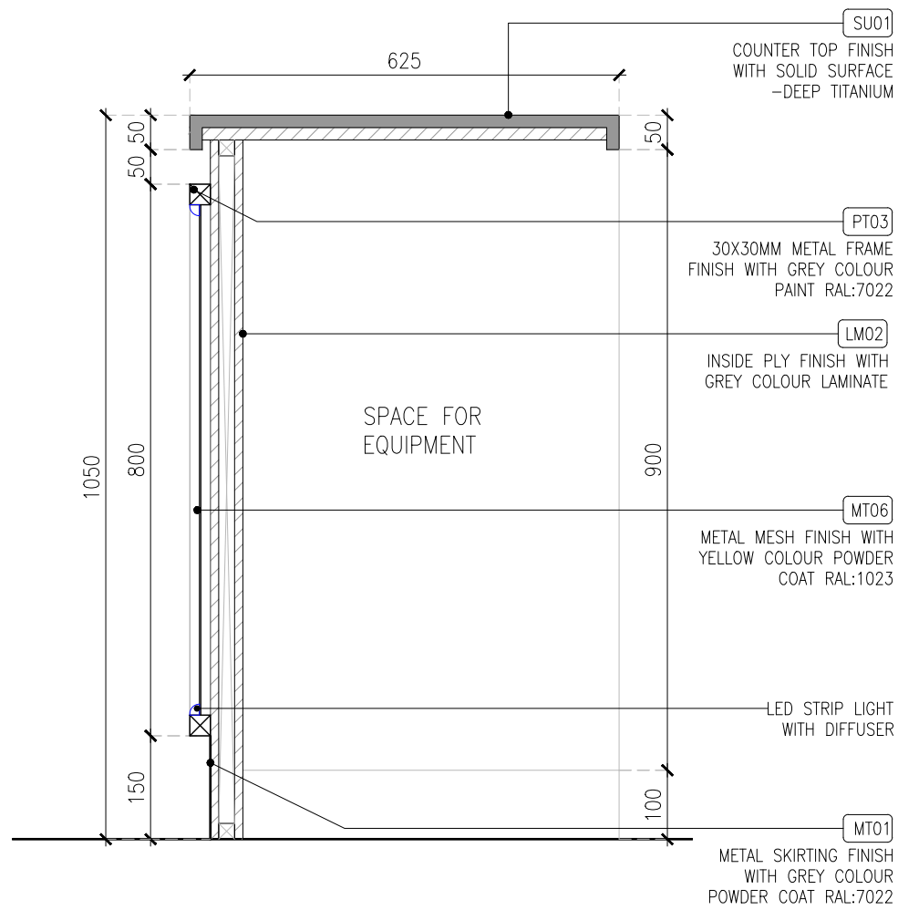
01 SECTION -01 04DE-411B 1:10
