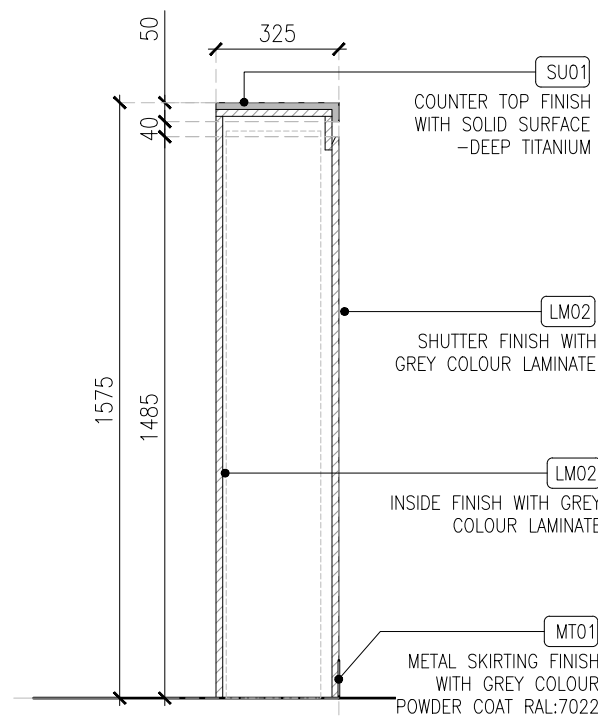
04 SECTION -04 04DE-411B 1:10
