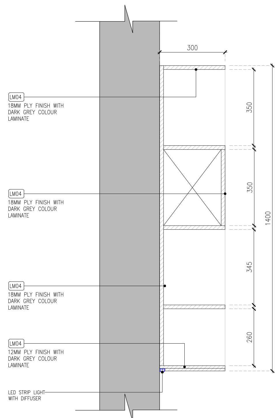
02 SECTION-02 04DE-412B 1:10
