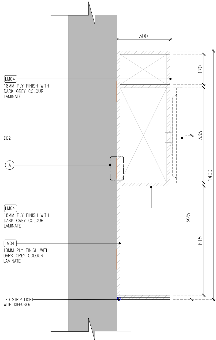
01 SECTION-01 04DE-412B 1:10
