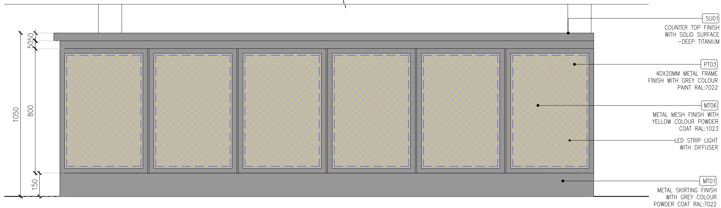
01 ELEVATION -01 04DE-411A 1:15
