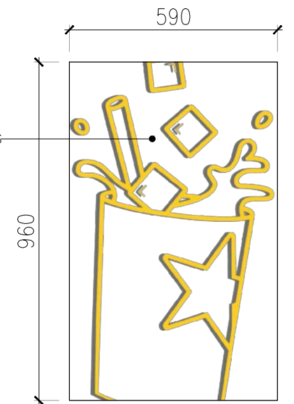
DETAIL-A(SCALE 1:15)
