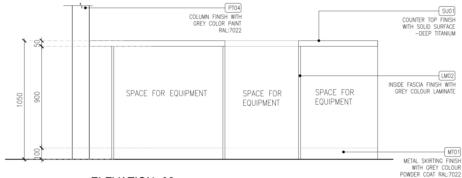
02 ELEVATION -02 04DE-411A 1:15
