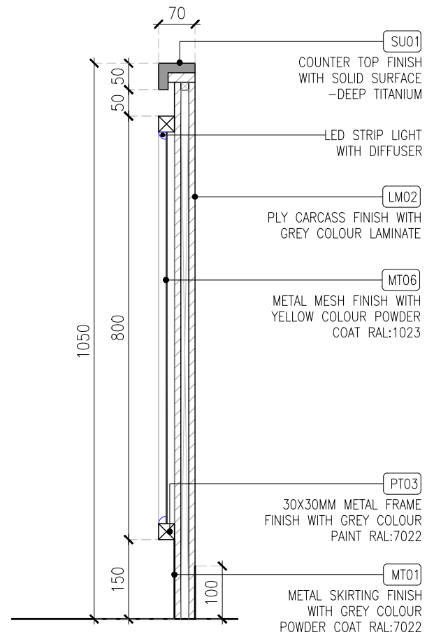
02 SECTION -02 04DE-411B 1:10
