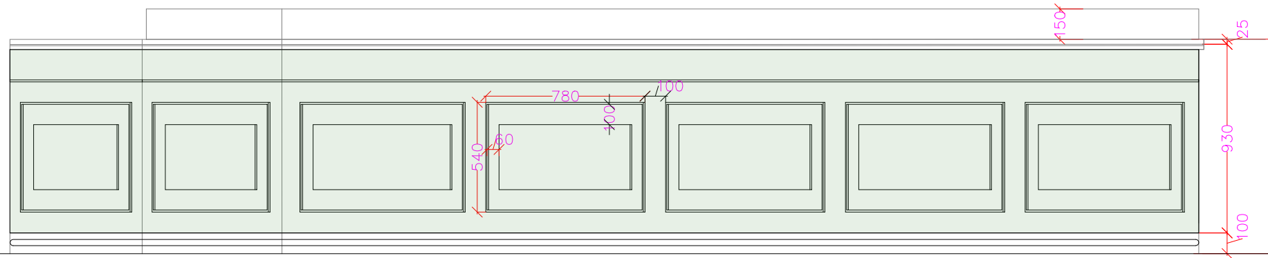
ELEVATION B
