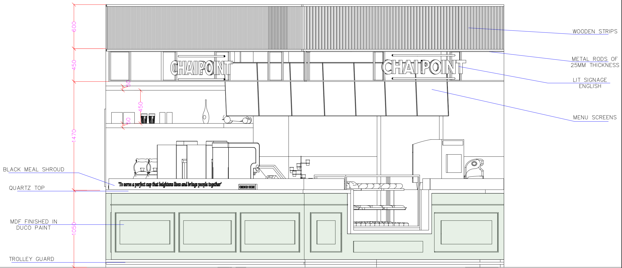
ELEVATION A
