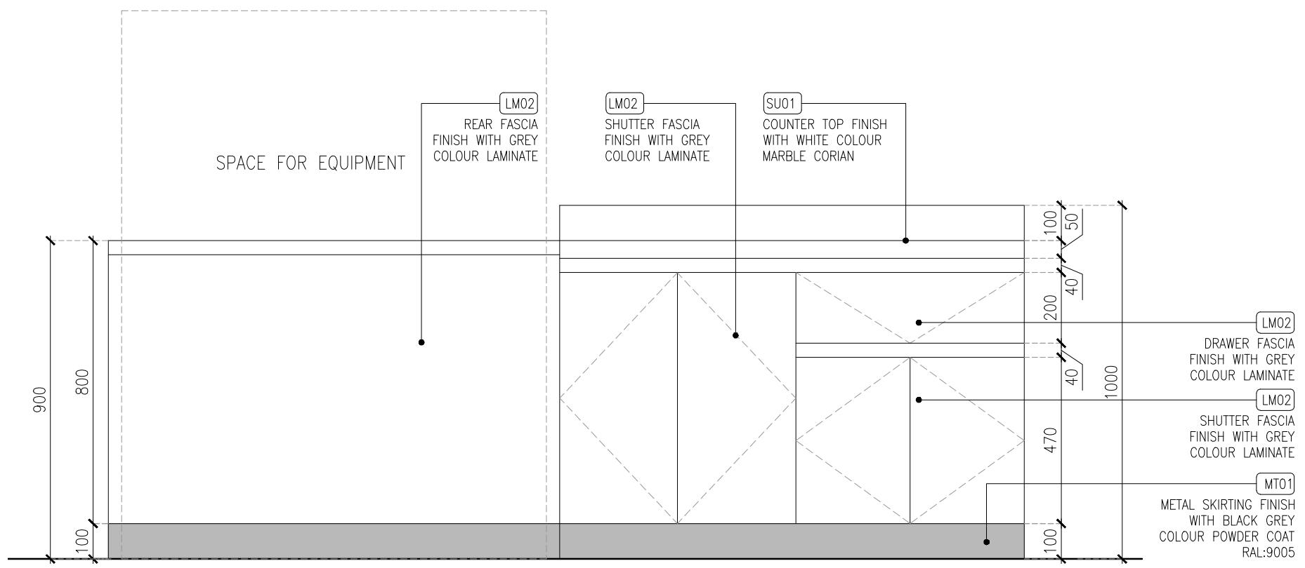
01 ELEVATION -03 04DE-402 1:15
