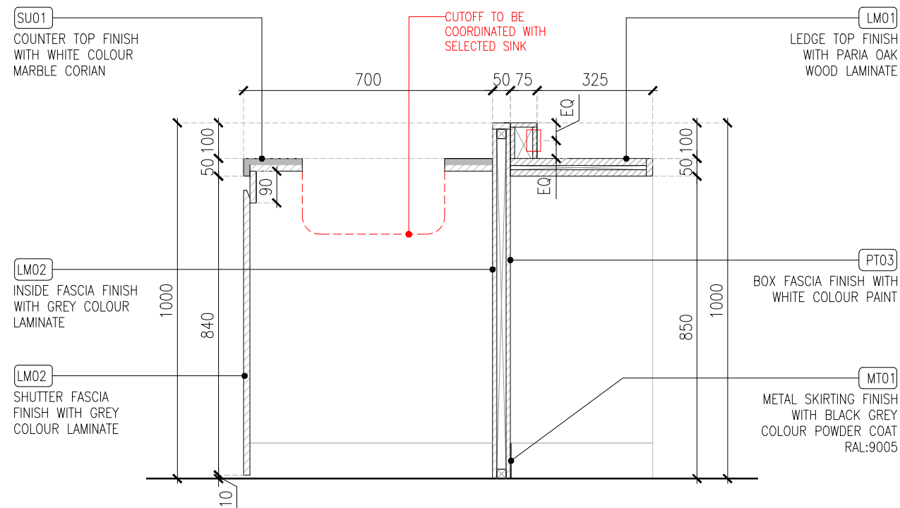
03 SECTION -04 04DE-403 1:15
