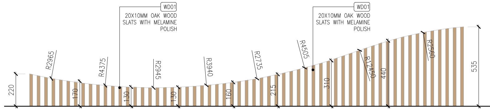
DETAIL-A(OAK WOOD SLATS)
