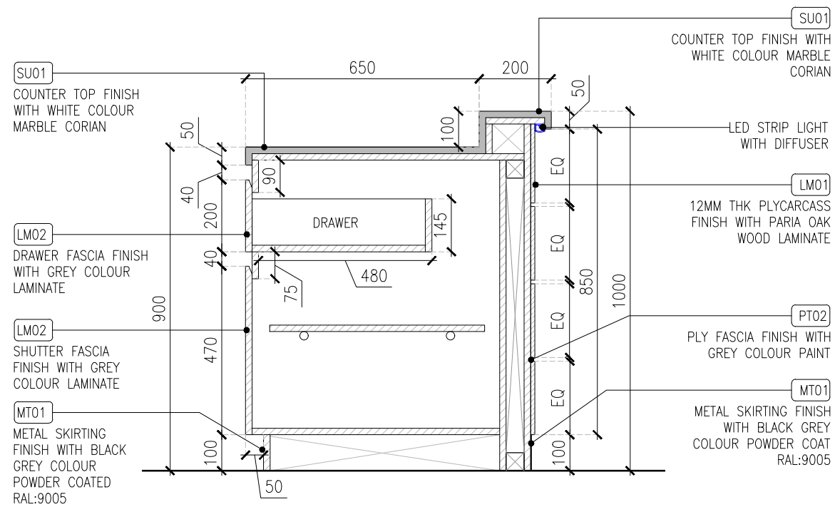
01 SECTION -02 04DE-403 1:15
