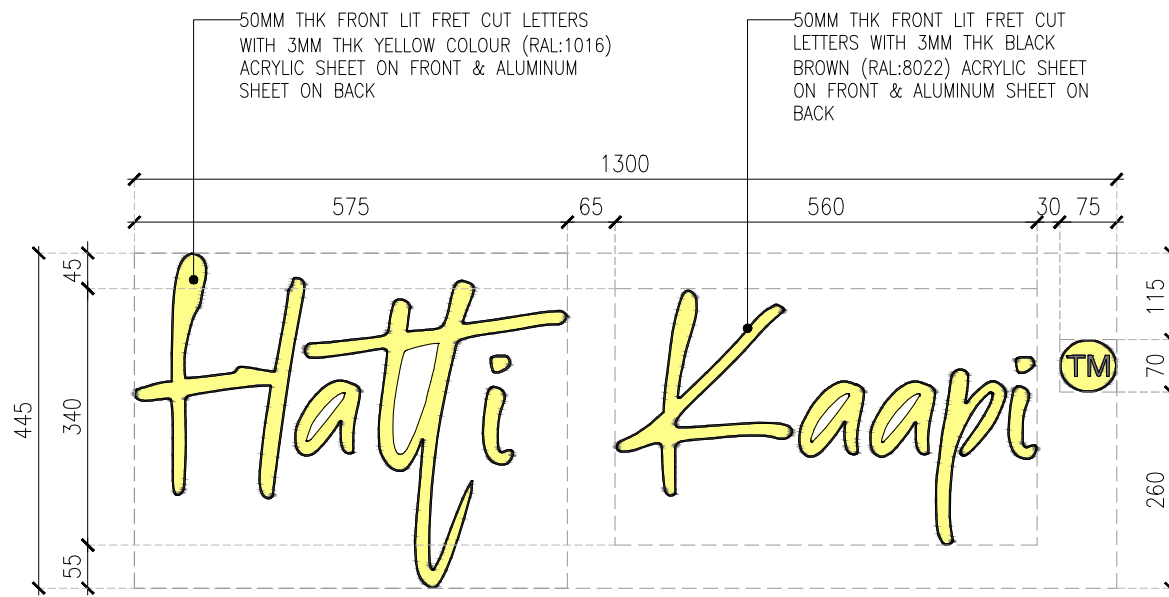
01 LIT SIGNAGE-01 (SG01)(2NOS) 04DE-413 1:10
