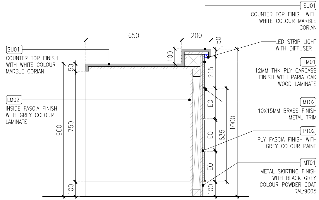
02 SECTION -03 04DE-403 1:15
