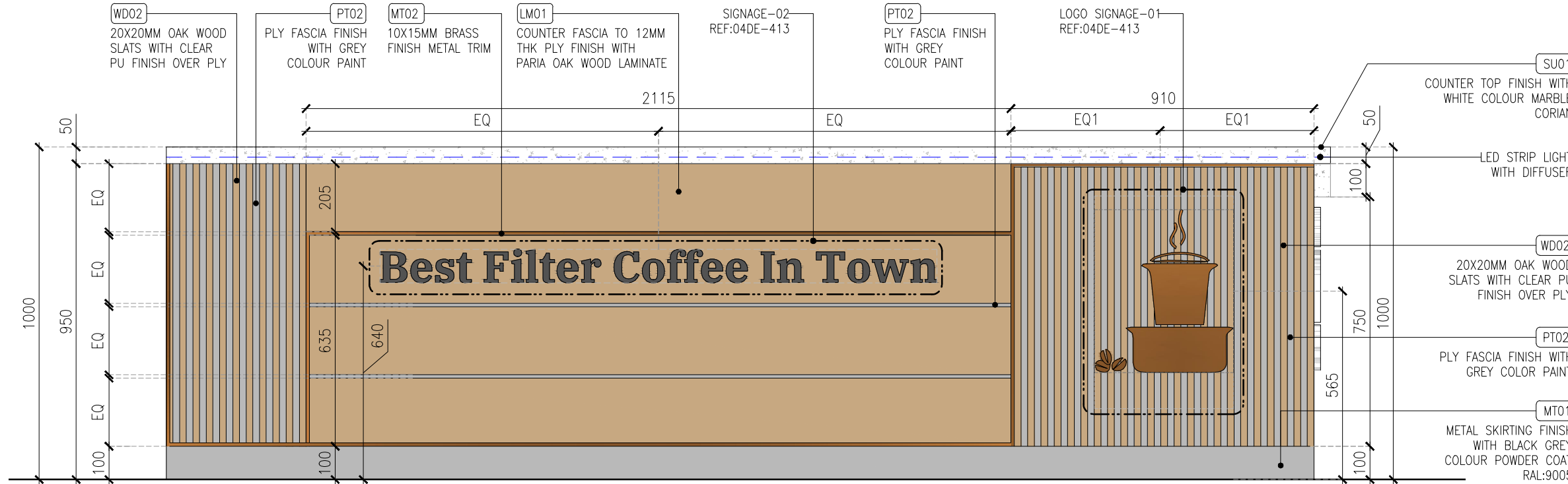
01 ELEVATION -01 04DE-401 1:15
