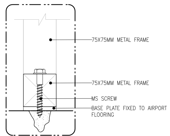
DETAIL-B (SCALE 1:5)
