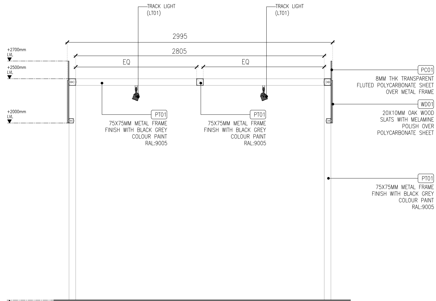
SECTION - A(SCALE 1:25)
