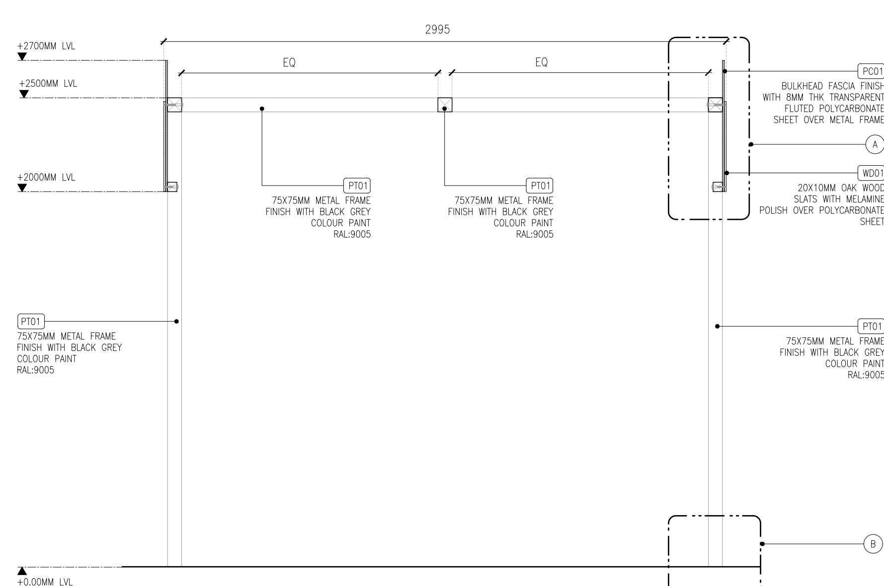
01 SECTION - 01 04DE-412 1:20
