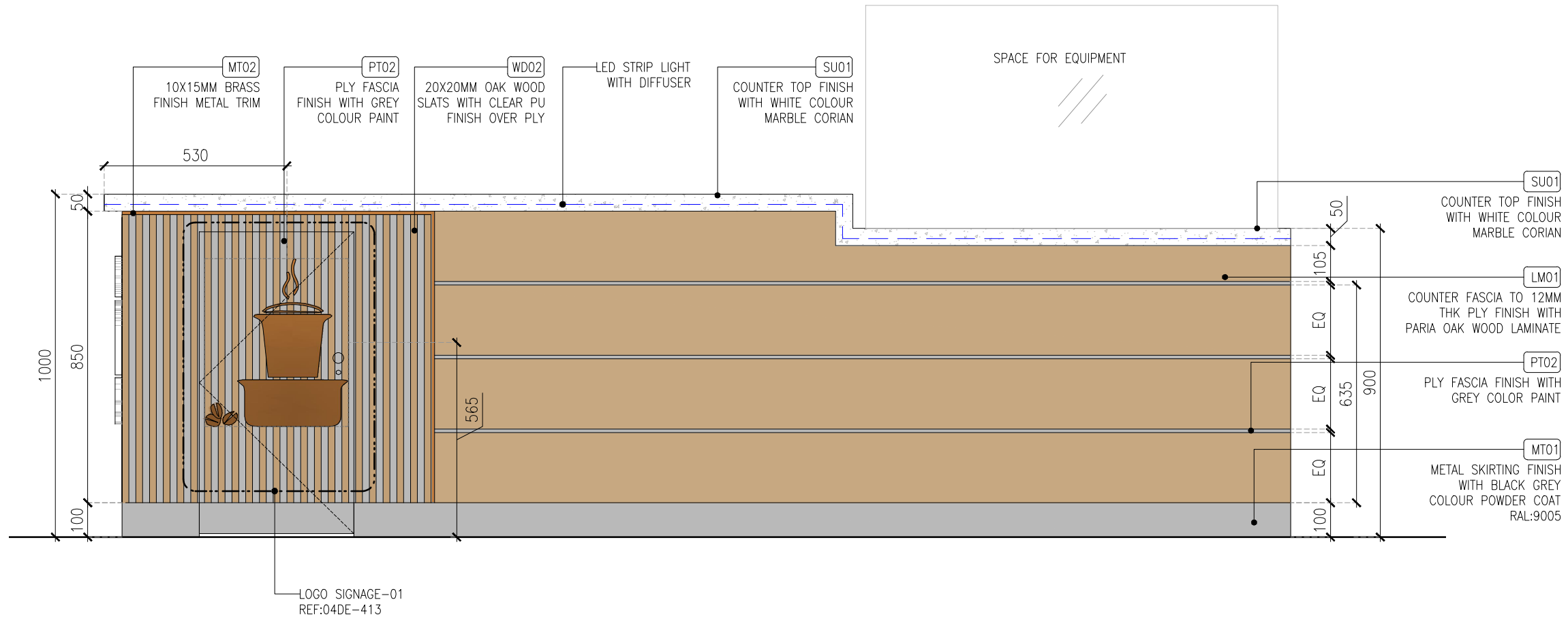
01 ELEVATION -01 04DE-401 1:15
