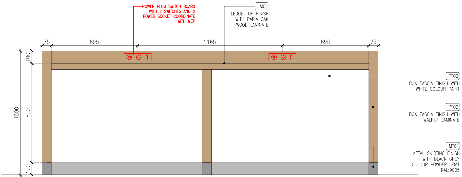
02 ELEVATION -04 04DE-402 1:15
