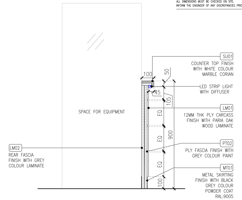
03 SECTION -01 04DE-402 1:15
