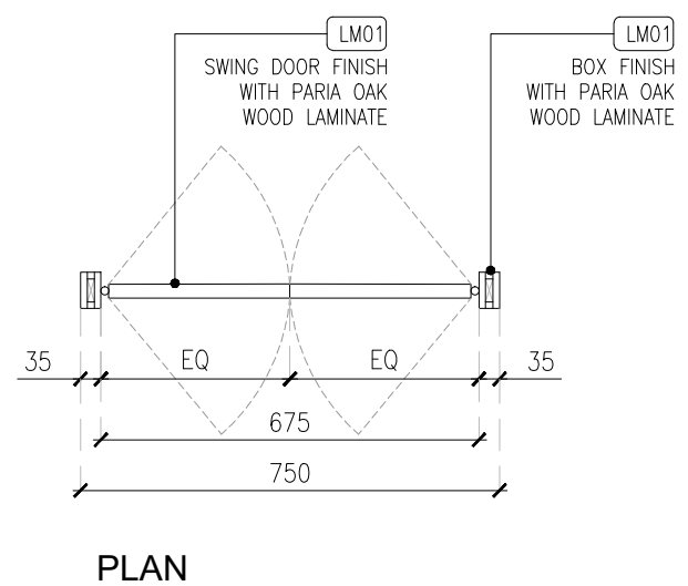
02 J04-SWING DOOR DETAIL-A 03IL-302 1:15
