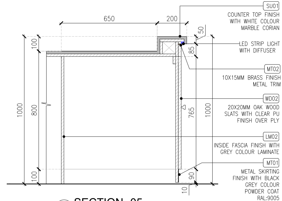
04 SECTION -05 04DE-403 1:15
