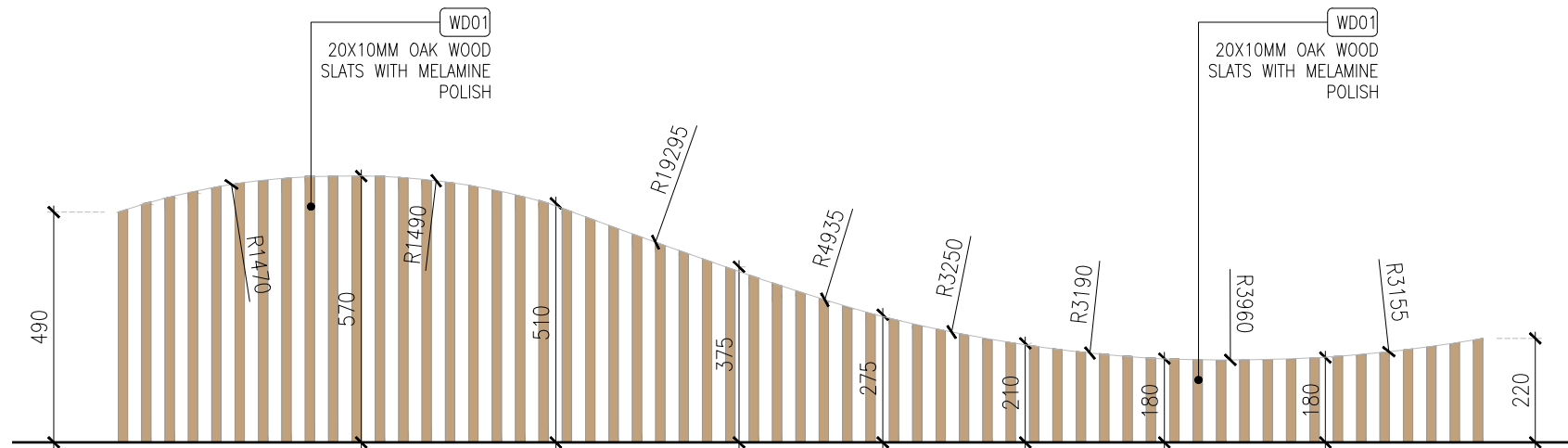
DETAIL-A(OAK WOOD SLATS)
