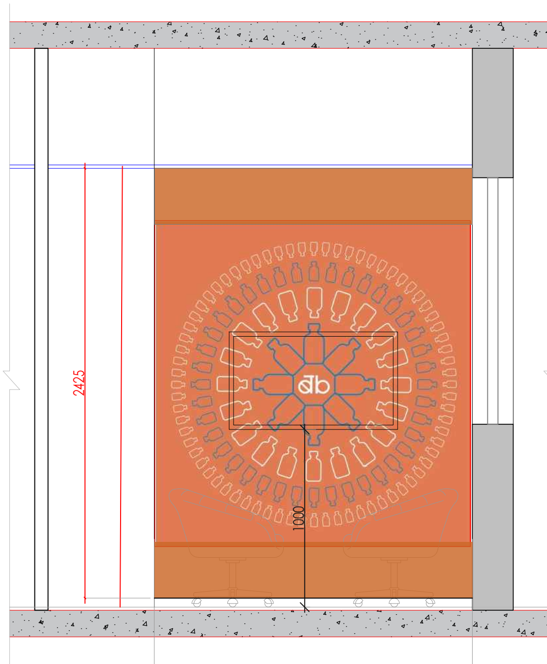
ELEVATION -09
