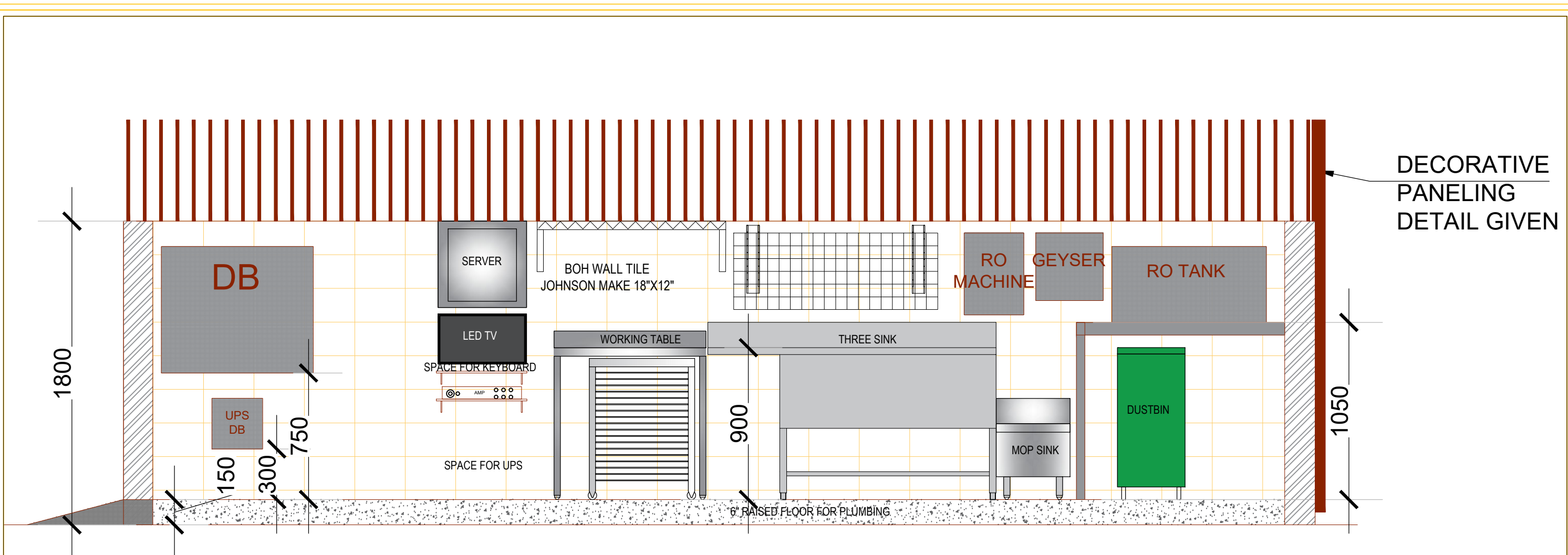
ELEVATION D-D
