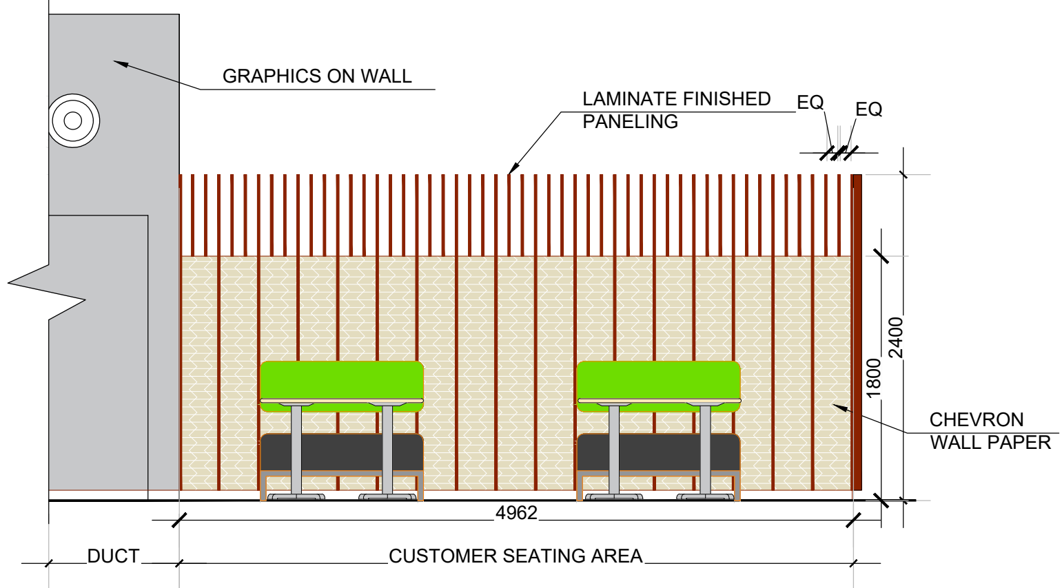
ELEVATION A-A
