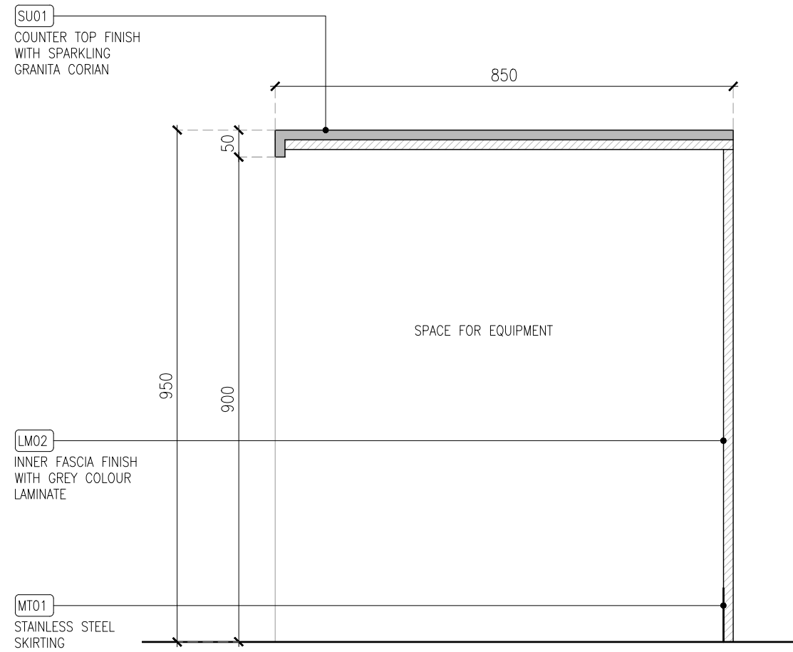
01 SECTION-01 04DE-404 1:10
