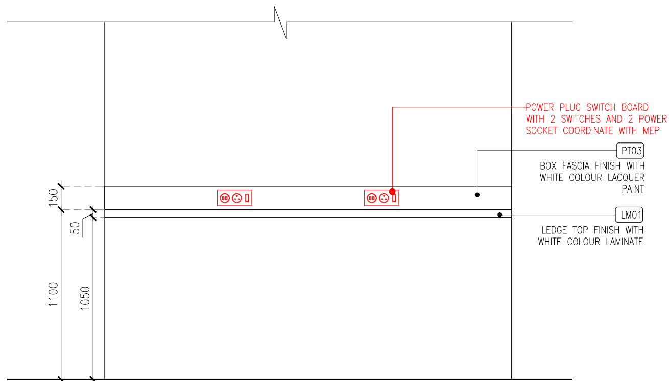
01 ELEVATION -01 04DE-410 1:25
