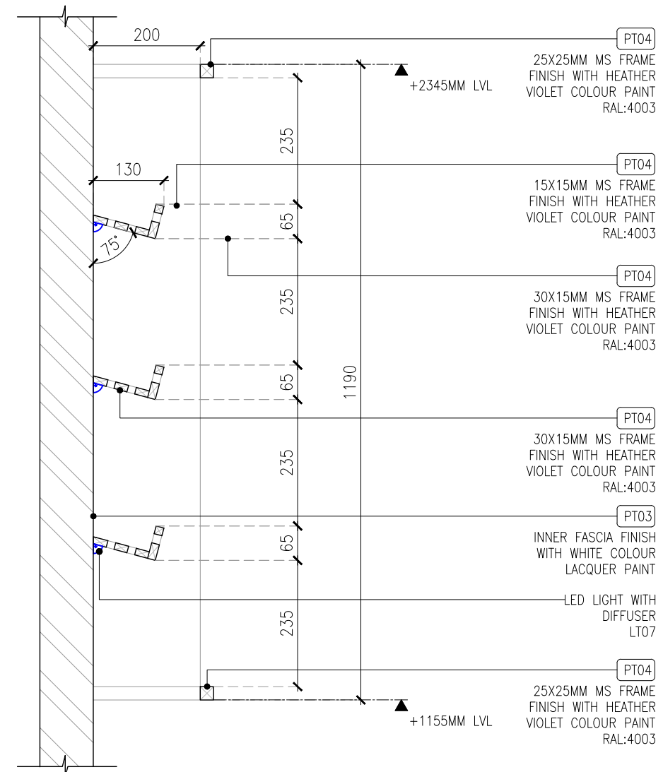
SECTION -A (SCALE 1:10)
