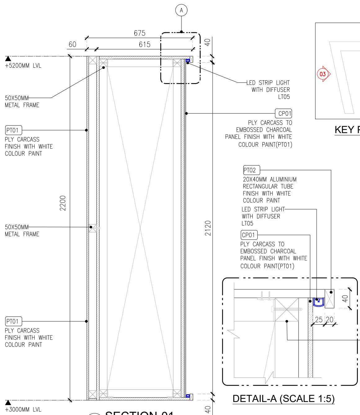
04 SECTION-01 04DE-406 1:15
