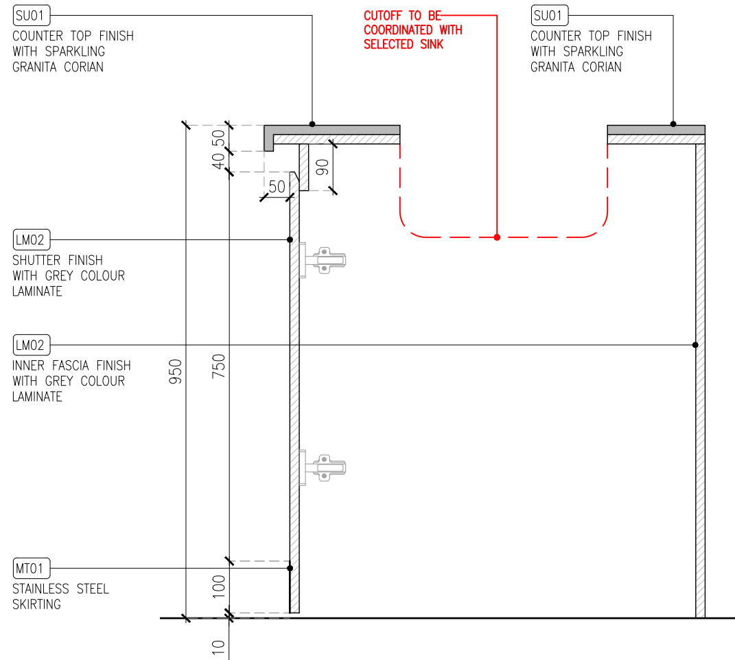
02 SECTION-02 04DE-404 1:10
