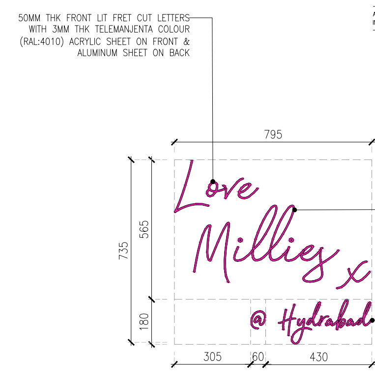
03 LIT SIGNAGE-03 (SG03) 04DE-415 1:15
