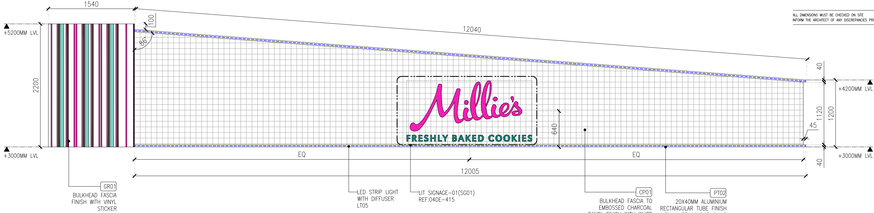
01 ELEVATION -01 04DE-406 1:40
