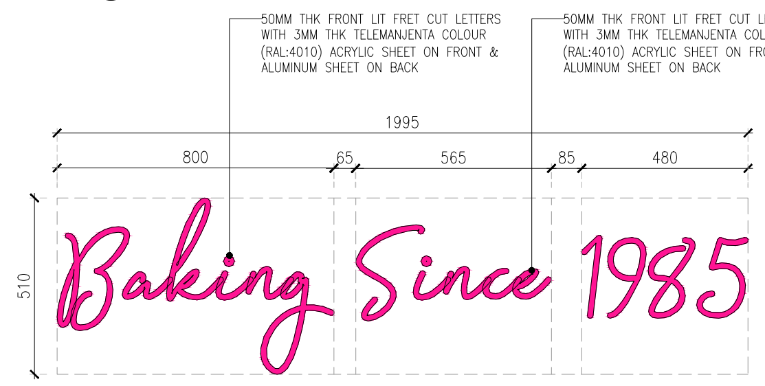
04 LIT SIGNAGE-04(SG04) 04DE-415 1:15
