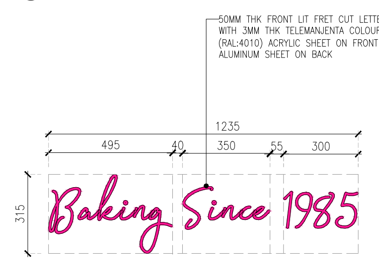
05 LIT SIGNAGE-05(SG05) 04DE-415 1:15
