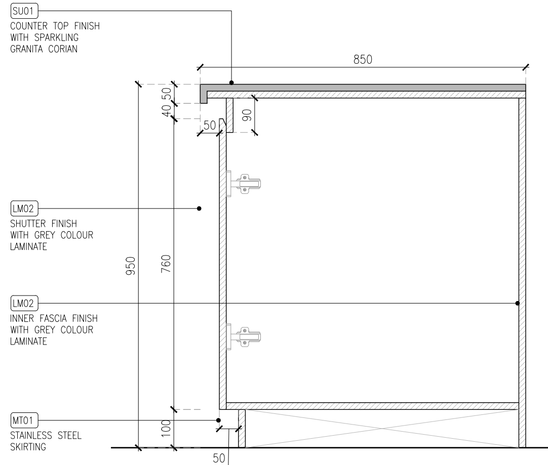
03 SECTION-03 04DE-404 1:10
