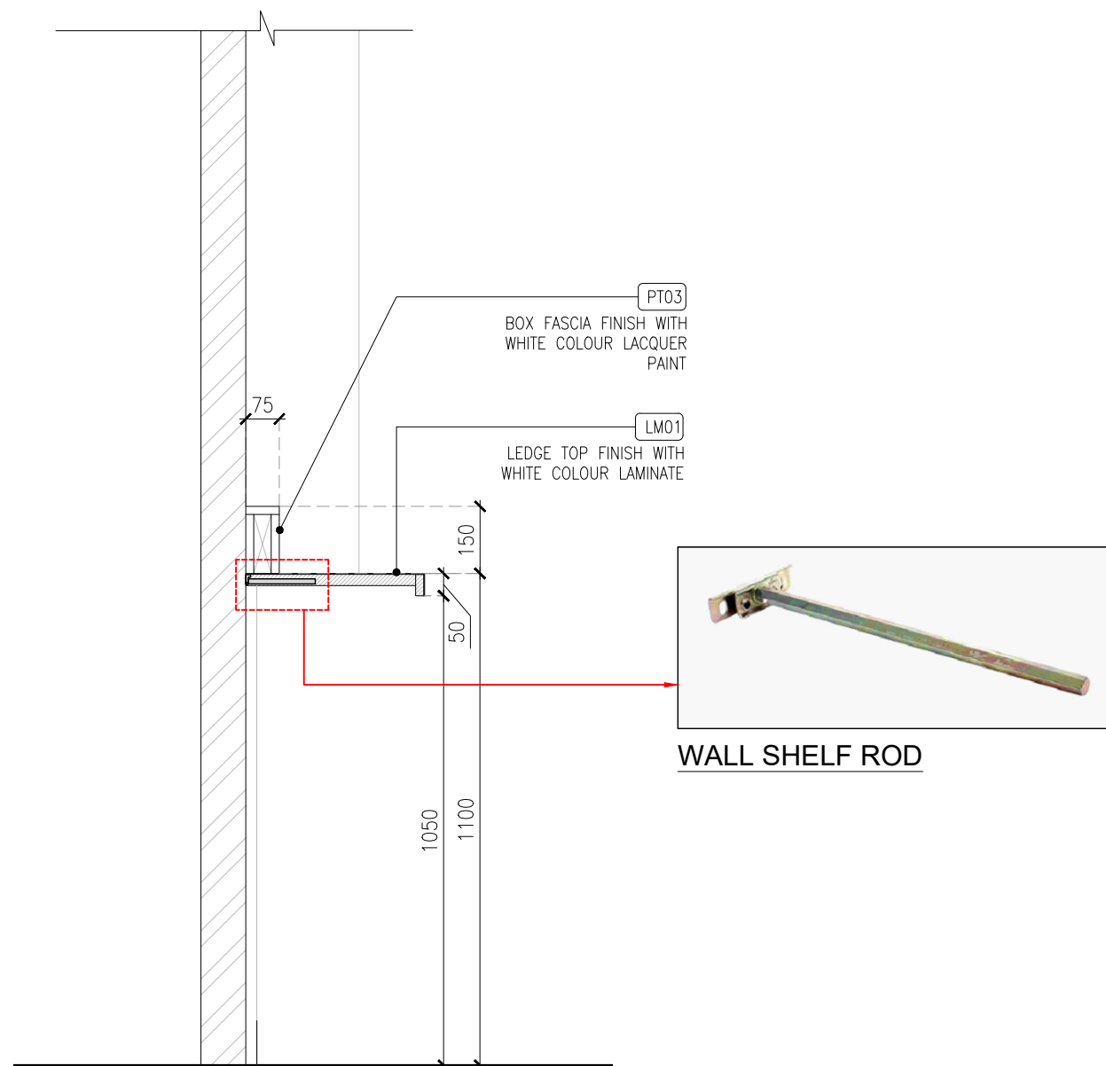
03 SECTION-01 04DE-410 1:15
