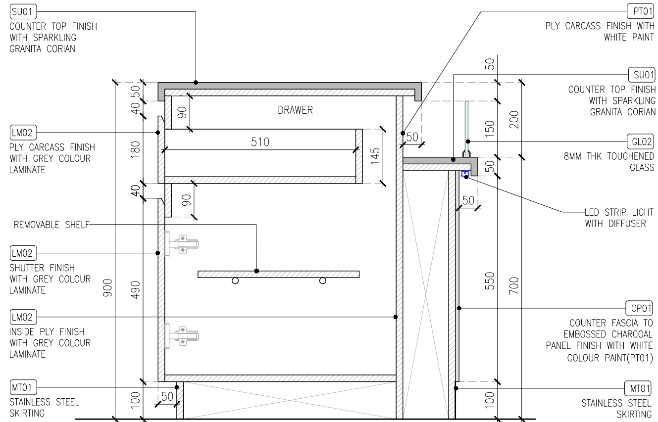
01 SECTION -01 04DE-402 1:10
