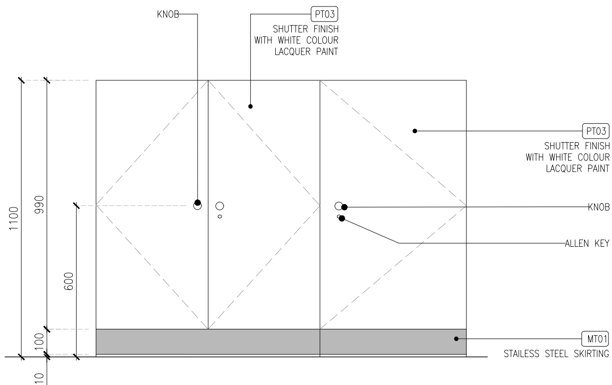
ELEVATION-01(SCALE 1:15)
