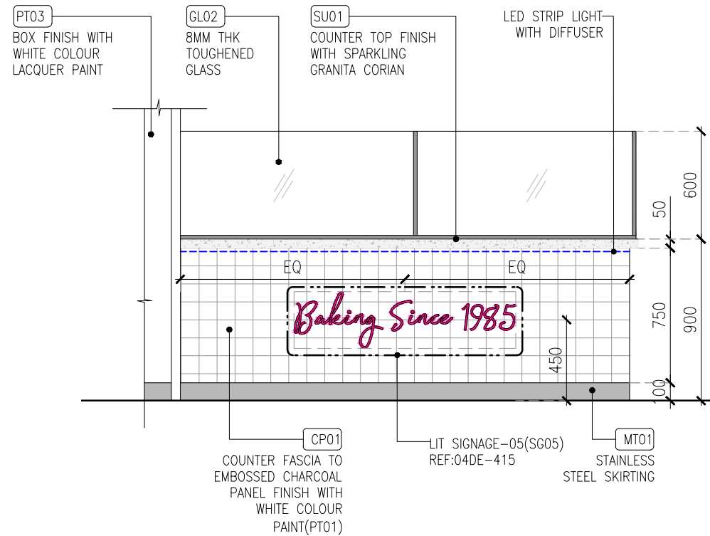
02 ELEVATION-02 04DE-401 1:30
