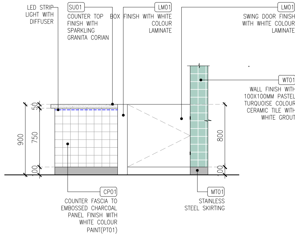
03 ELEVATION-03 04DE-401 1:30
