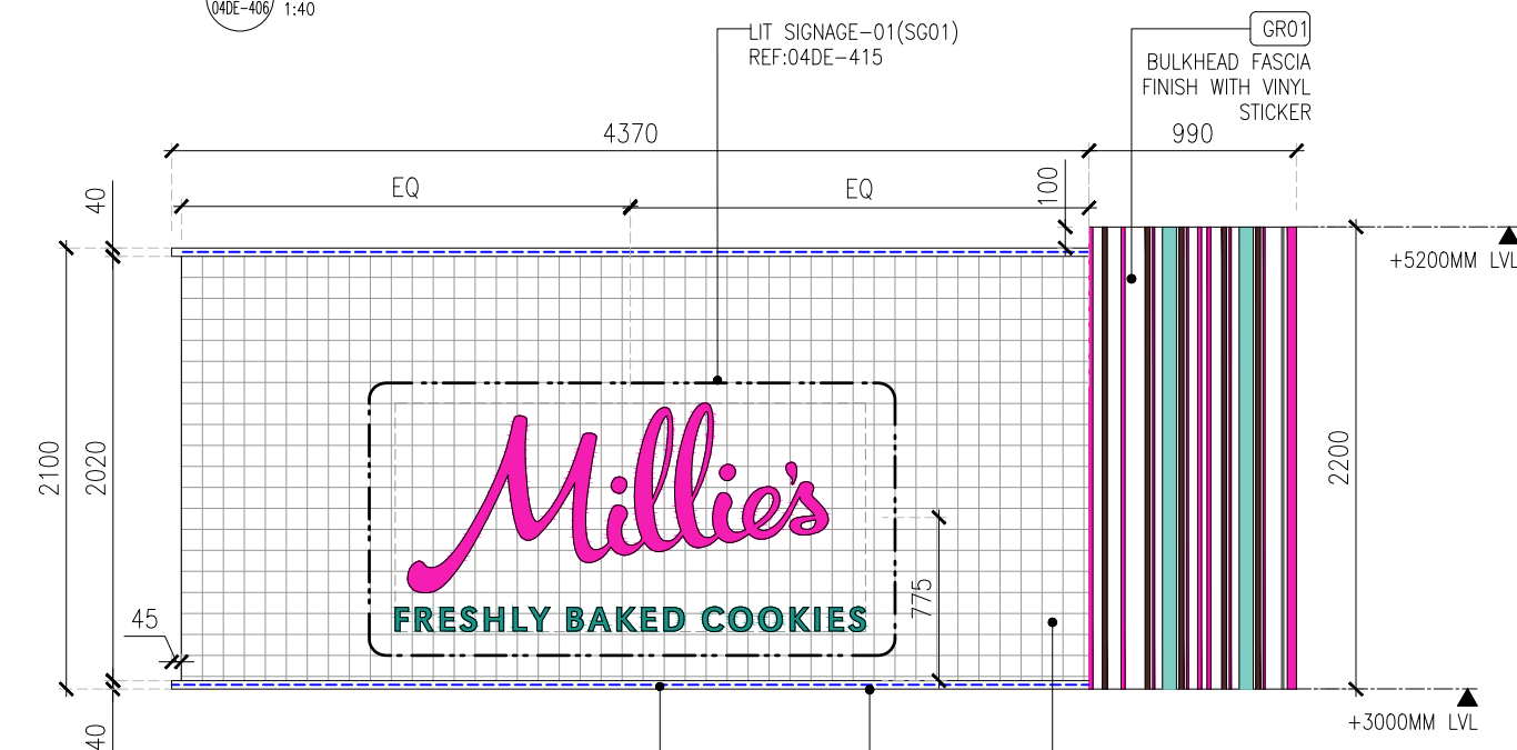
02 ELEVATION -02 04DE-406 1:40
