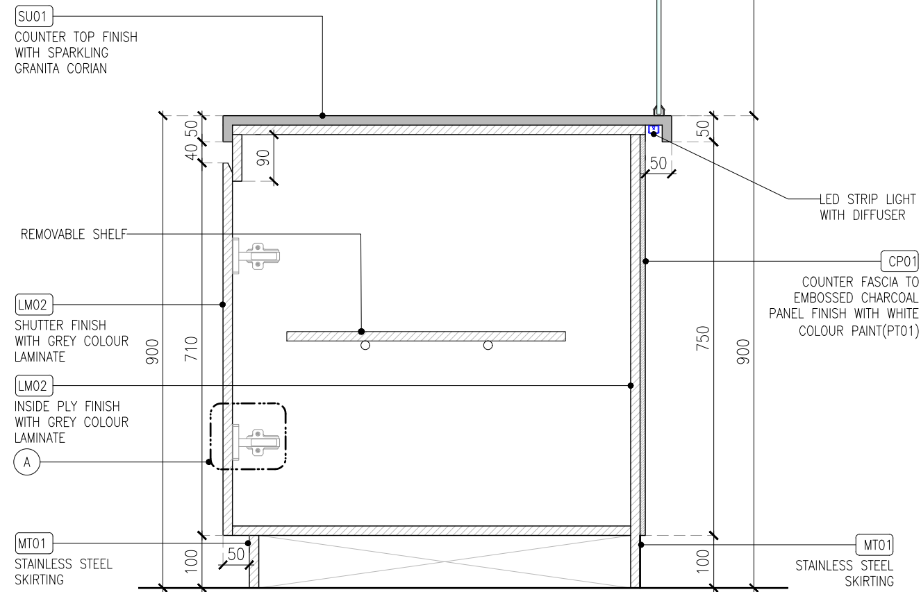
02 SECTION -02 04DE-402 1:10
