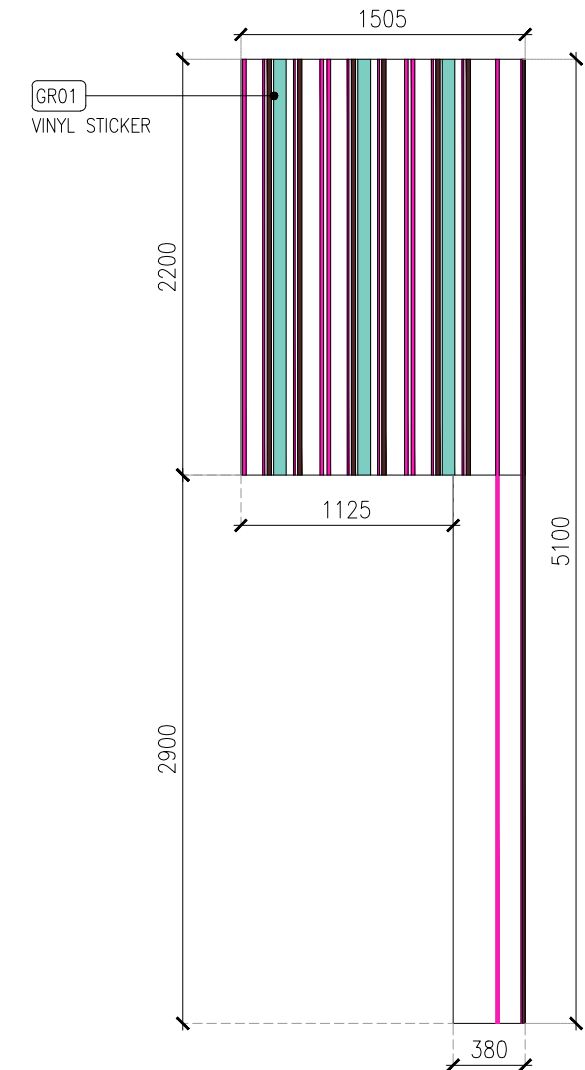
DETAIL-A(SCALE 1:40)
