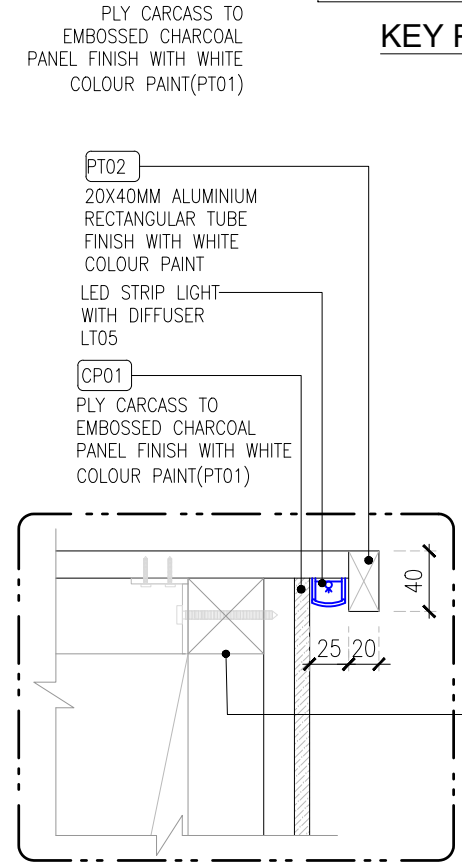
DETAIL-A (SCALE 1:5)
