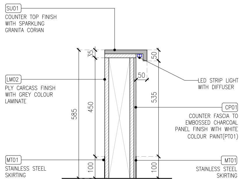
03 SECTION -03 04DE-402 1:10
