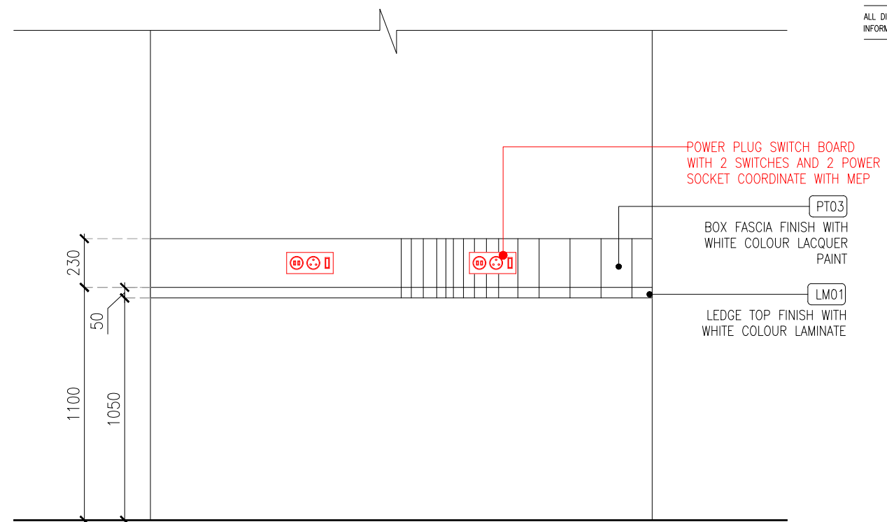
02 ELEVATION -02 04DE-410 1:25
