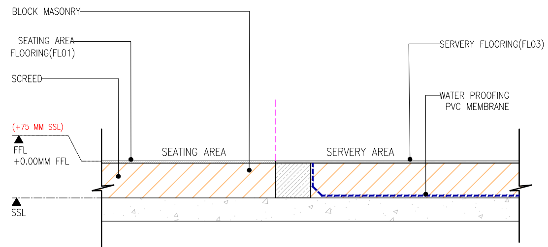
SECTION-A (SCALE 1:10)
