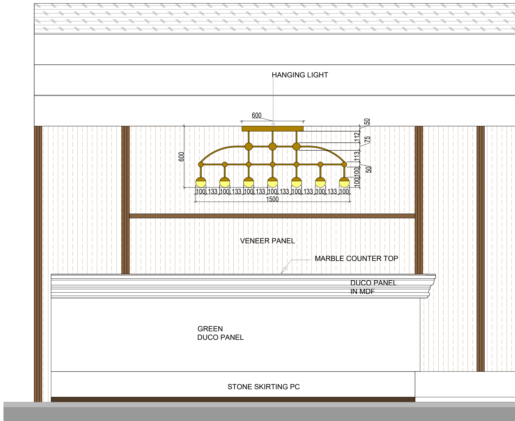
ELEVATION
